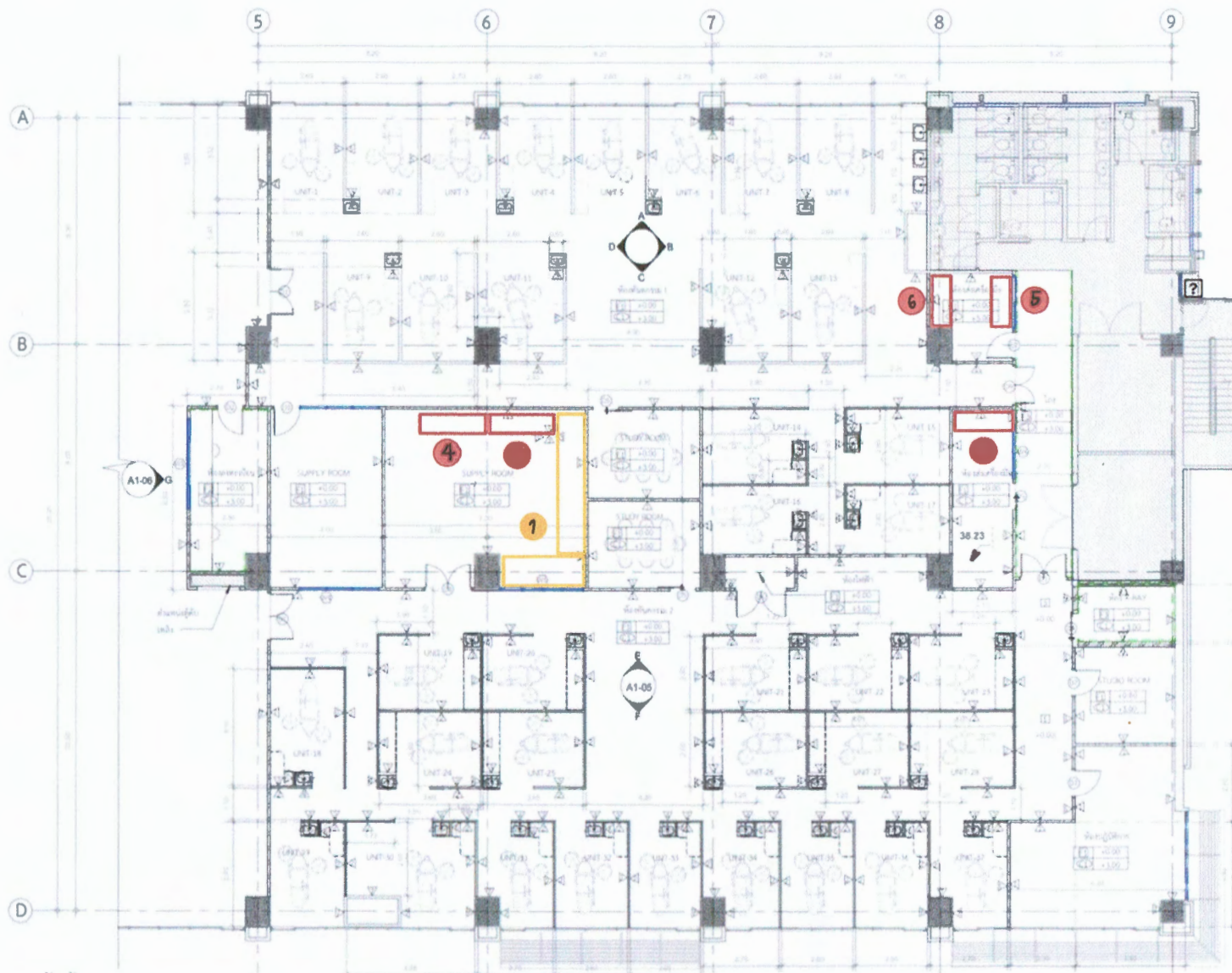
แปลนพื้นที่ 11 (แปลนขยายส่วนที่ปรับปรุง) 1:100
